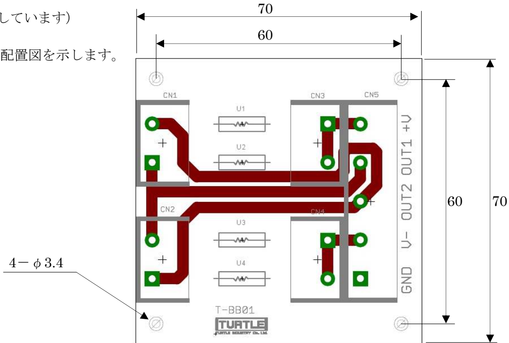
図1 配置図
