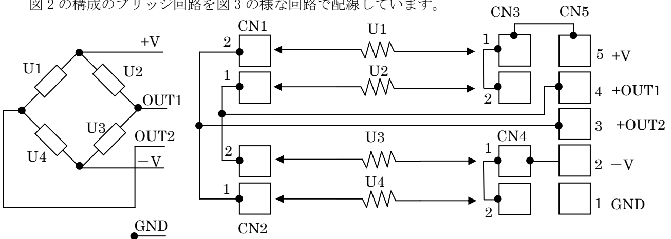
図2 回路構成
